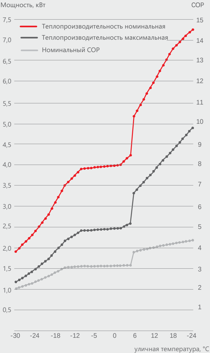
График теплопроизводительности и энергоэффективности RAS-25U2FVG-ND
