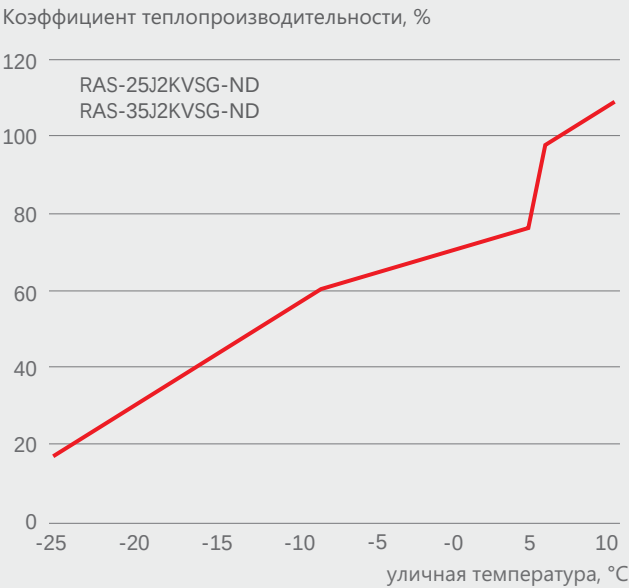
График зависимости теплопроизводительности от уличной температуры
