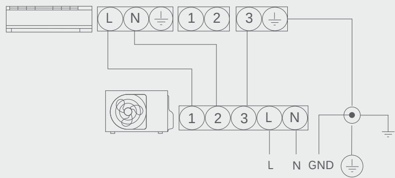
Электрическая схема
