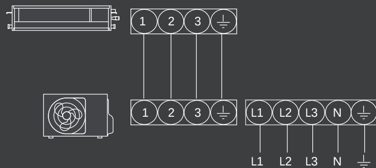
Электрическая схема
