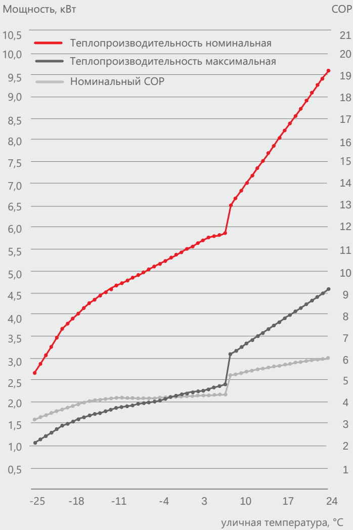
График теплопроизводительности и энергоэффективности RAS-10N4KVRG-EE
