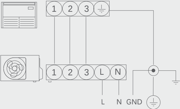
Электрическая схема (опциональная)
