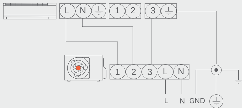
Электрическая схема
