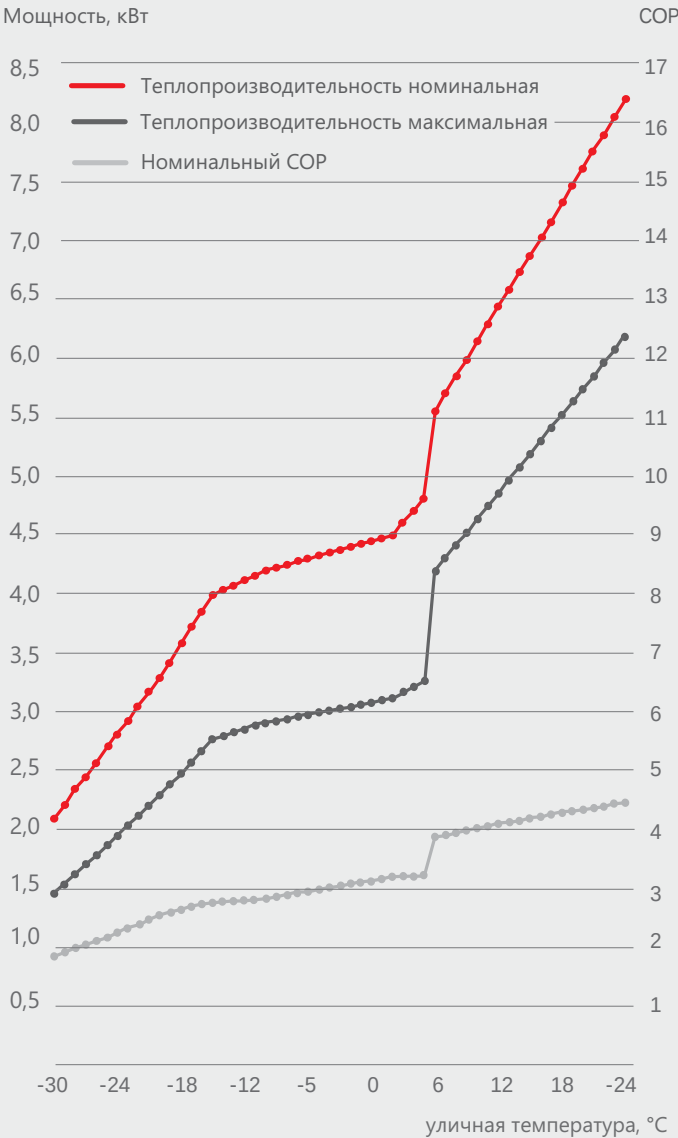
График теплопроизводительности и энергоэффективности RAS-35U2FVG-ND
