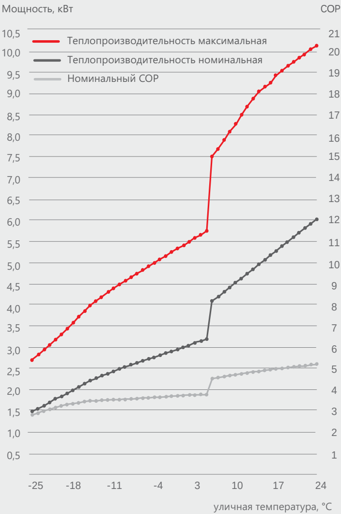
График теплопроизводительности и энергоэффективности RAS-25J2KVSG-ND
